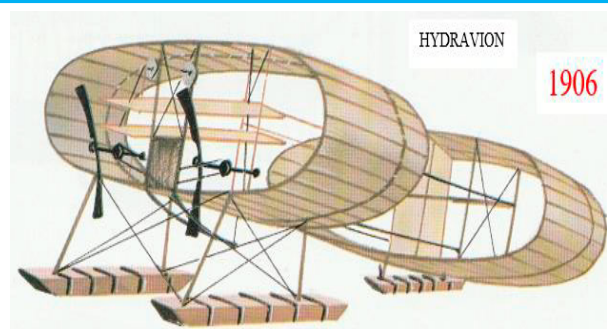
Blériot III France Moteur Antoinette 8 cylindres en V 25 CH Structure ; sapin, frêne revêtement toile
