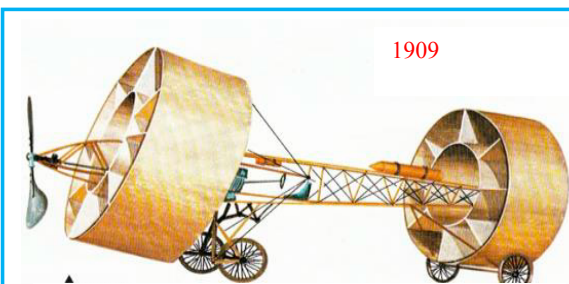
Givaudan France Moteur Antoinette 8 cylindres en V 40 CH Longueur 5,79 Structure tubes métalliques et bois ,revêtement toile
